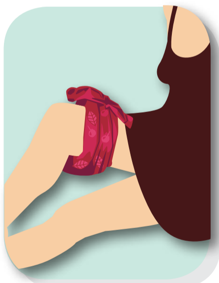
Genou Cuisse
